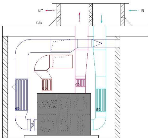
boven: schematisch aanzicht van de luchtgroep met bovenaansluiting van de kanalen recht: verfijnde detaillering van de trap
